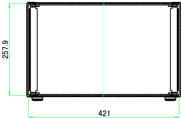
A-A ( 1 : 6.5 )
